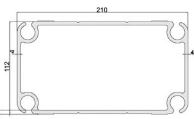
Profilo principale
