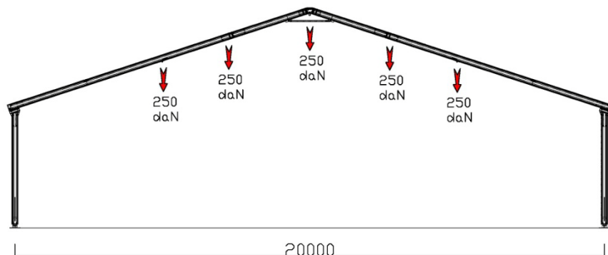
ARCATA INTERMEDIA
